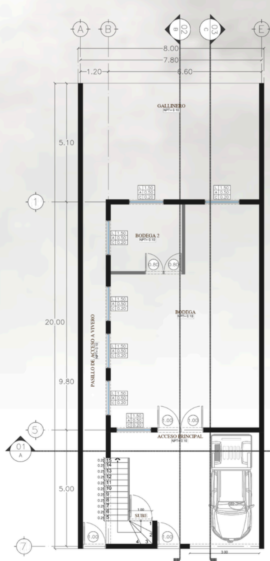
PLANTA ARQUITETONICA NIVEL PRINCIPAL
